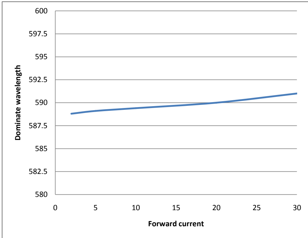
Fig. 1-13 Forward current vs. Dominate wavelength 正向电流与主波长特性曲线 (Ts=25°C)
