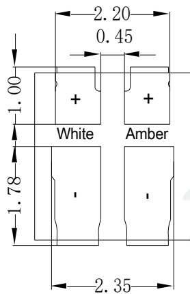
Fig.1-3 Bottom View 背面视图
