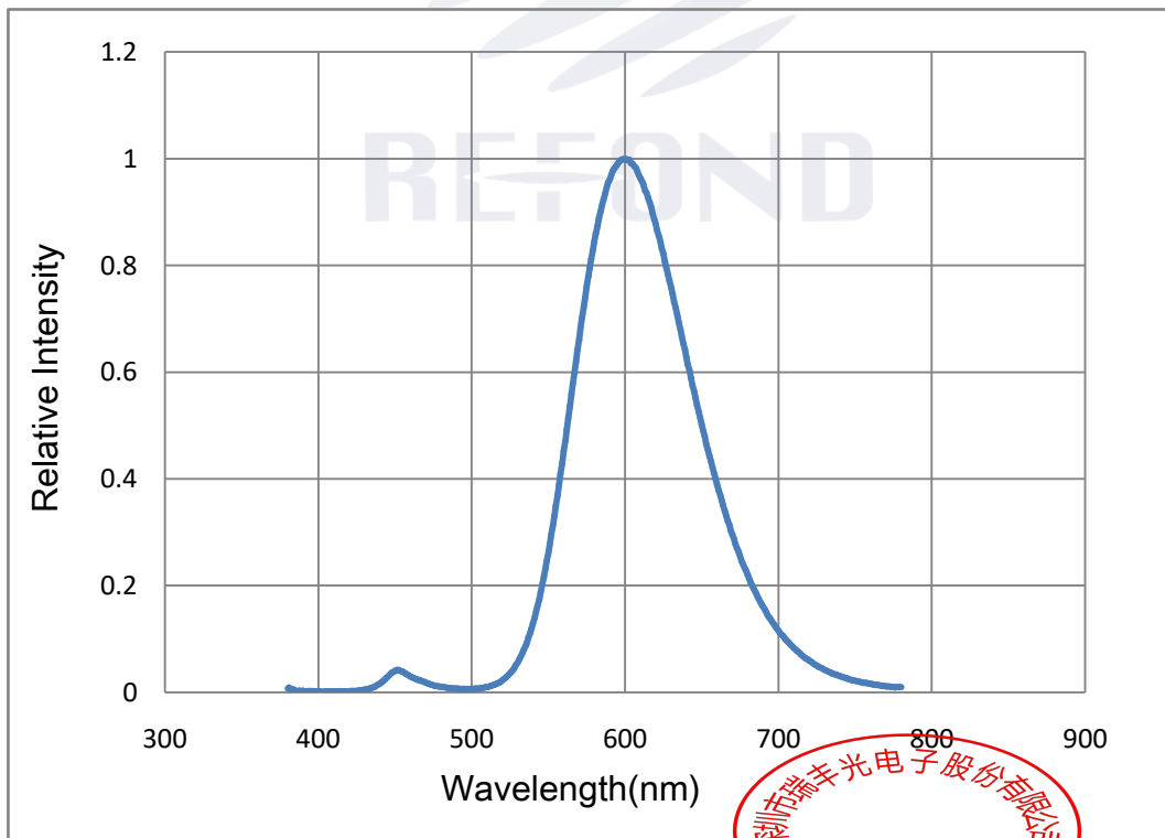
Fig. 1-14 Spectrum Distribution(Amber)光谱分布特性曲线 (琥珀光)
