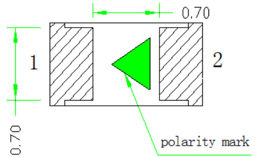
Fig.1-2 Bottom view 背面视图
