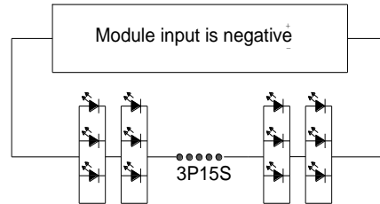
Fig.2-2ED Module connection 模組電性圖
