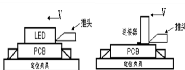
Fig 7-2 Push & Pull Test Method 推拉力测试方法
