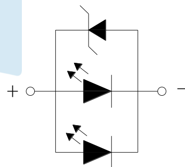
Fig.1-4 Polarity 极性
