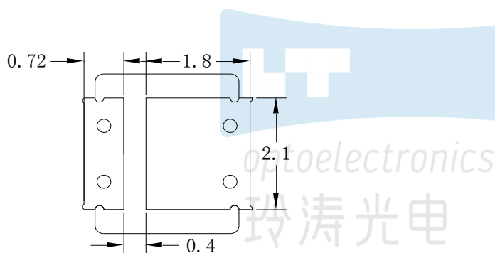
Fig.1-1 Top view 正面视图
