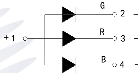
Fig.1-4 Polarity 极性
